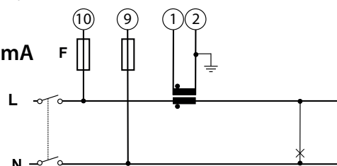
Connessione da 1 TA
